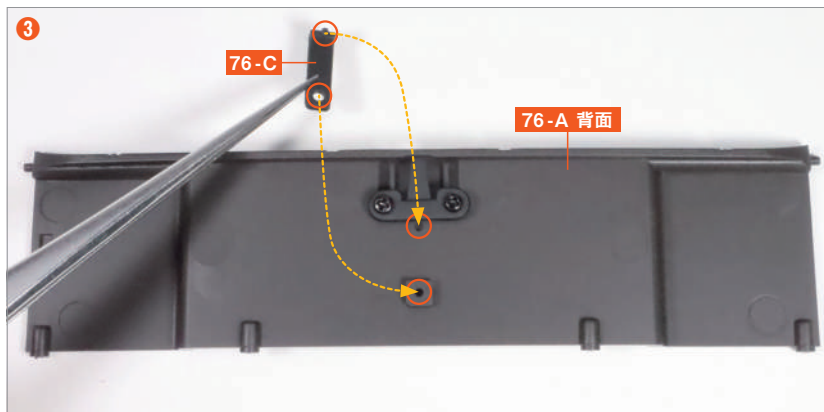
將鎖扣支架 76-C 的螺絲孔和小突起, 分別對準 76-A 背面的螺絲孔和小孔進行組裝。
